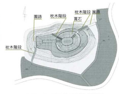
▲古墳整備工事（墳丘整備）平面図
