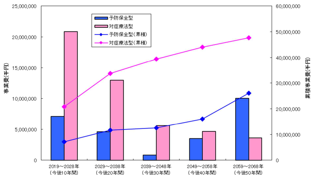
今後 50 年間の従来手法と長寿命化修繕計画との将来経費予測
