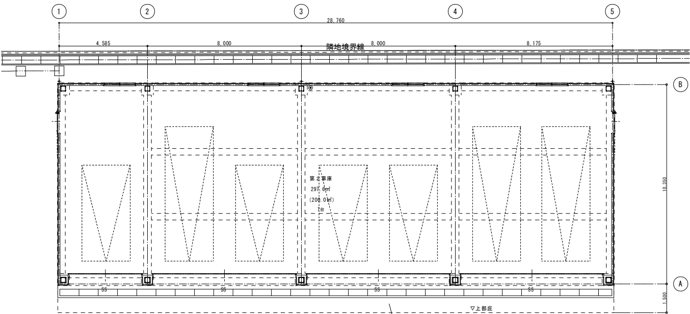
第2車庫平面図 S=1:100 グレーティング必要
