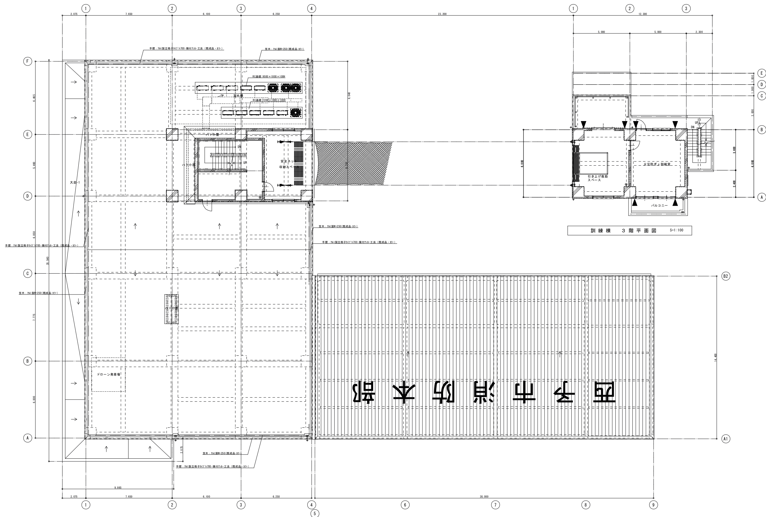
庁舎 3 階平面図 S=1:100
