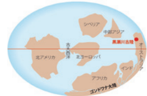
4 億年前の大陸の分布図
