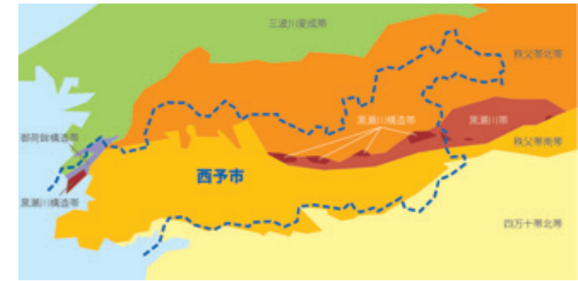
西予市周辺の地層の分布図
