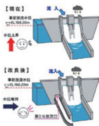
改良工事に伴う調節量の変化
